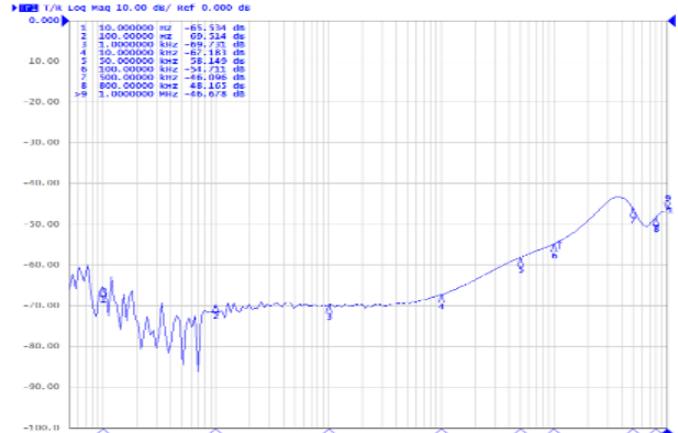
PSRR
