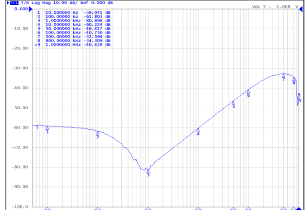
PSRR
