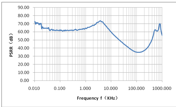
PSRR
